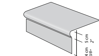
Gradone Lineare + Alzata 32,5x60 13"x24" Step + Stair "riser" Stufe + "Setztstufe" Treppe Nez de marche + "Contremarche" escalier 126
