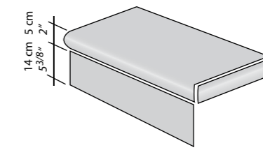
Gradone Angolare (DX / SX) + Alzata 32,5x60 13"x24" Corner step + Stair "riser" Eckstufe + "Setztstufe" Treppe Nez de marche angulaire + "Contremarche" escalier 293
